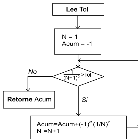
Figure 1.21: Diagrama de flujo correspondiente a la segunda solución.
