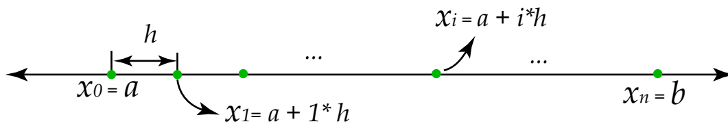
Figure 1.38: Partir el intervalo en n puntos.
