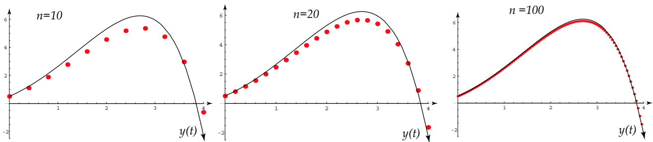
Figure 2.6: Aproximación con el método de Euler
