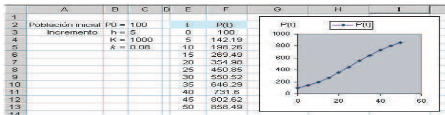
Figure 1.7: Curva obtenida para el modelo logístico de crecimiento de una población.
