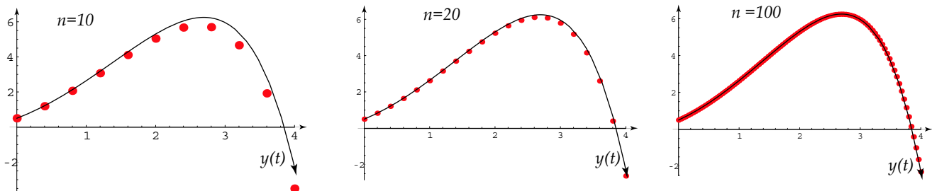
Figure 2.9: Método de Heun
