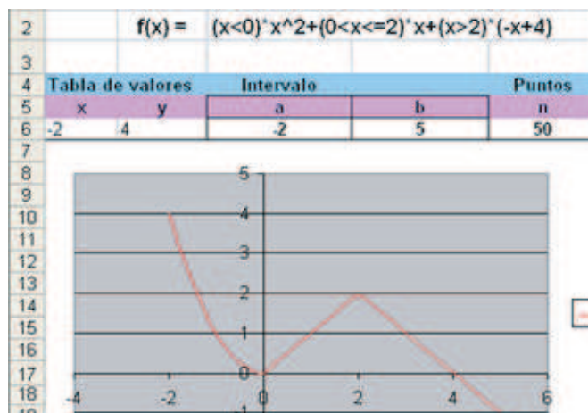
Figure 1.40: Función a trozos.
