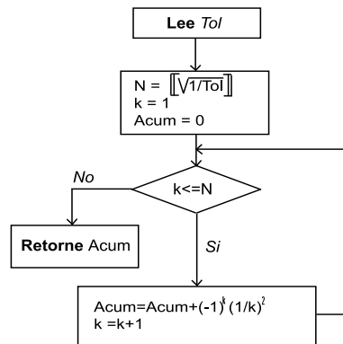
Figure 1.19: Diagrama de flujo correspondiente a la primera solución.
