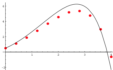
Figure 2.8: Método de Euler con n = 10
