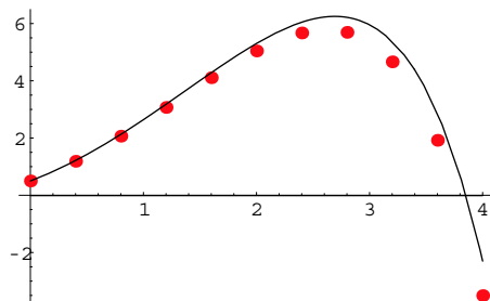
Figure 2.11: Método de Euler con n = 10
