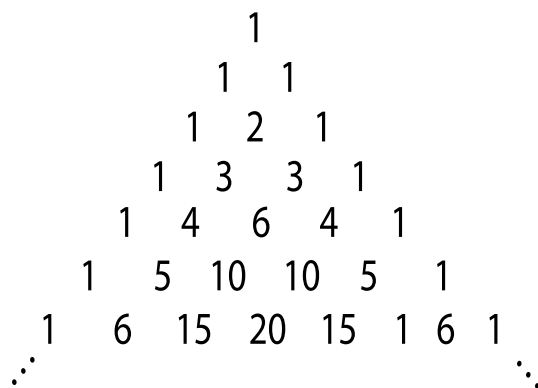
Figure 1.34: Triángulo de Pascal.
