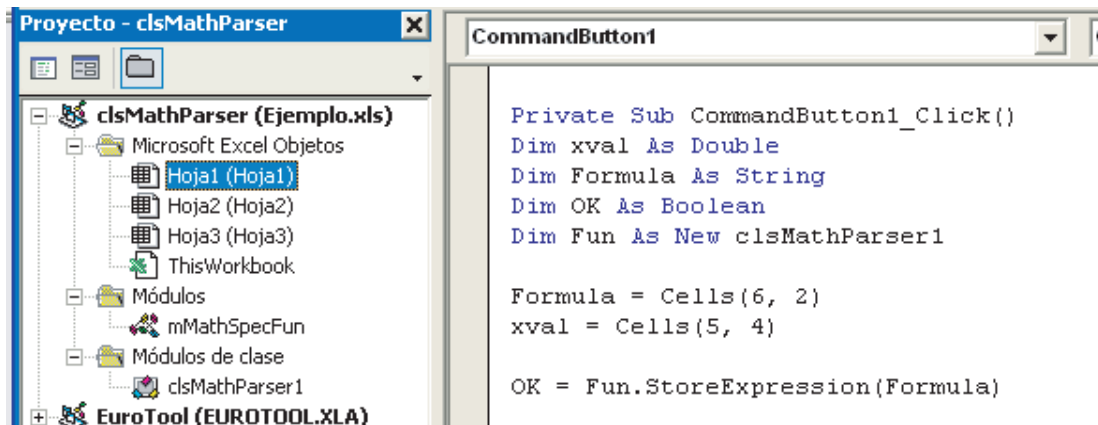
Figure 1.37: Editor VBA con los módulos.
